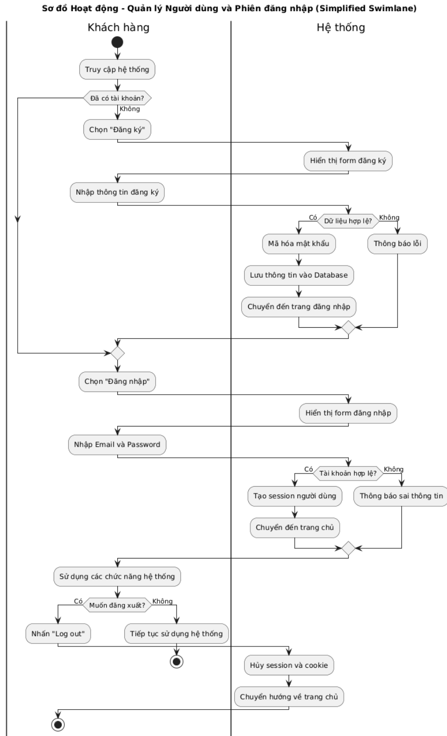
Hình 3.2 Sơ đồ Hoạt động – Quản lý người dùng và phiên đăng nhập
