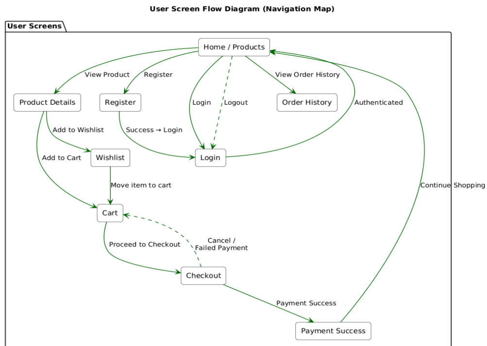
Hình 4.48 Sơ đồ liên kết các màn hình (Khách hàng)
