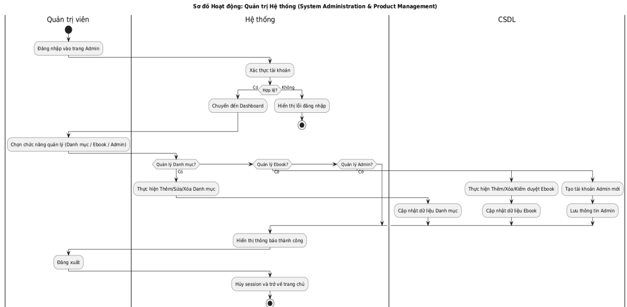
Hình 3.12 Sơ đồ hoạt động Quản trị hệ thống
