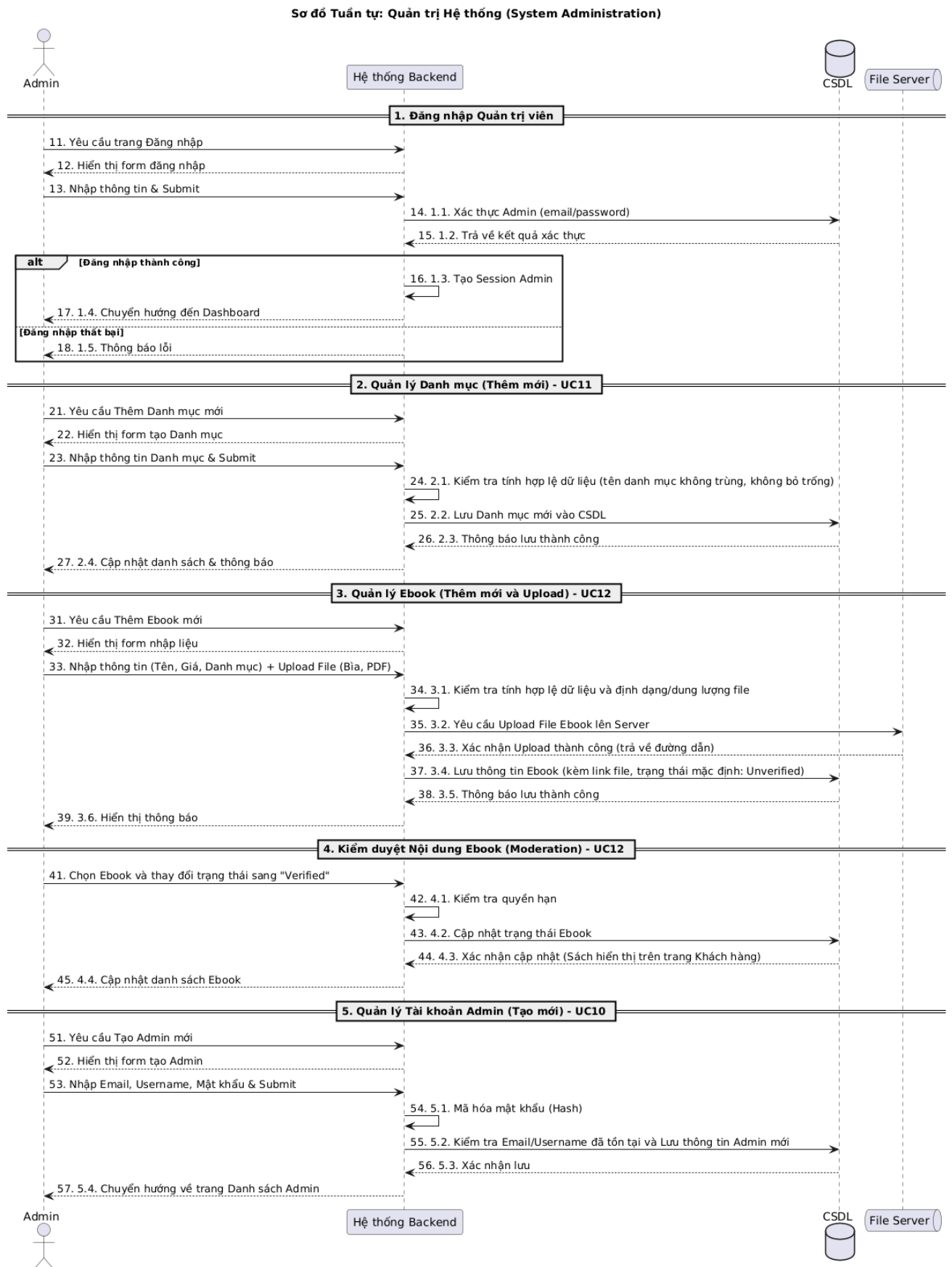
Hình 3.13 Sơ đồ tuần tự: Quản trị Hệ thống
