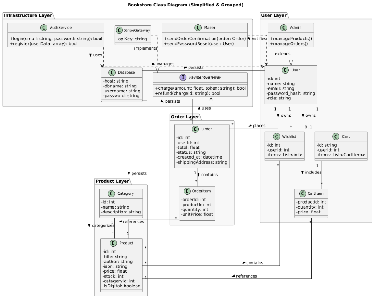
Hình 4.39 Class Diagram cơ sở dữ liệu
