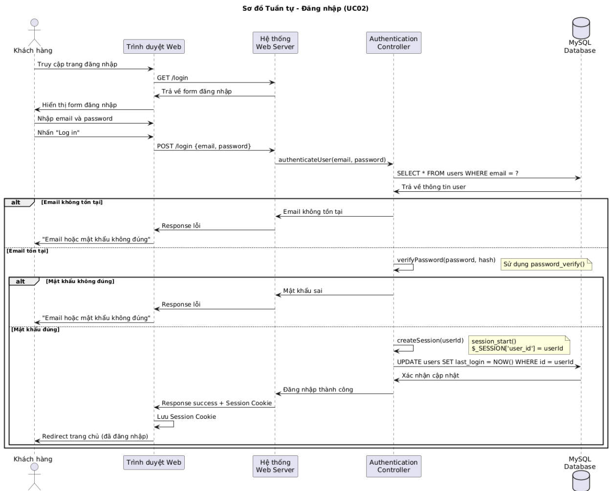
Hình 3.4 Sơ đồ tuần tự - Đăng nhập
