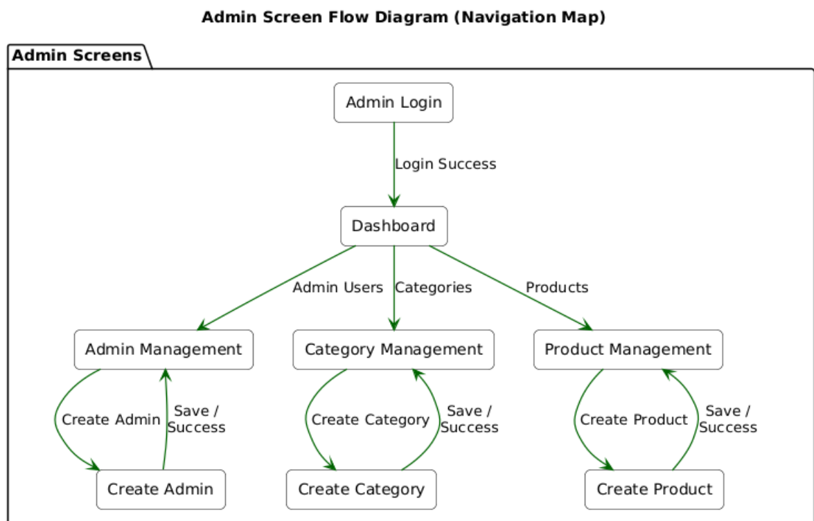
Hình 4.49 Sơ đồ liên kết các màn hình (Admin)
