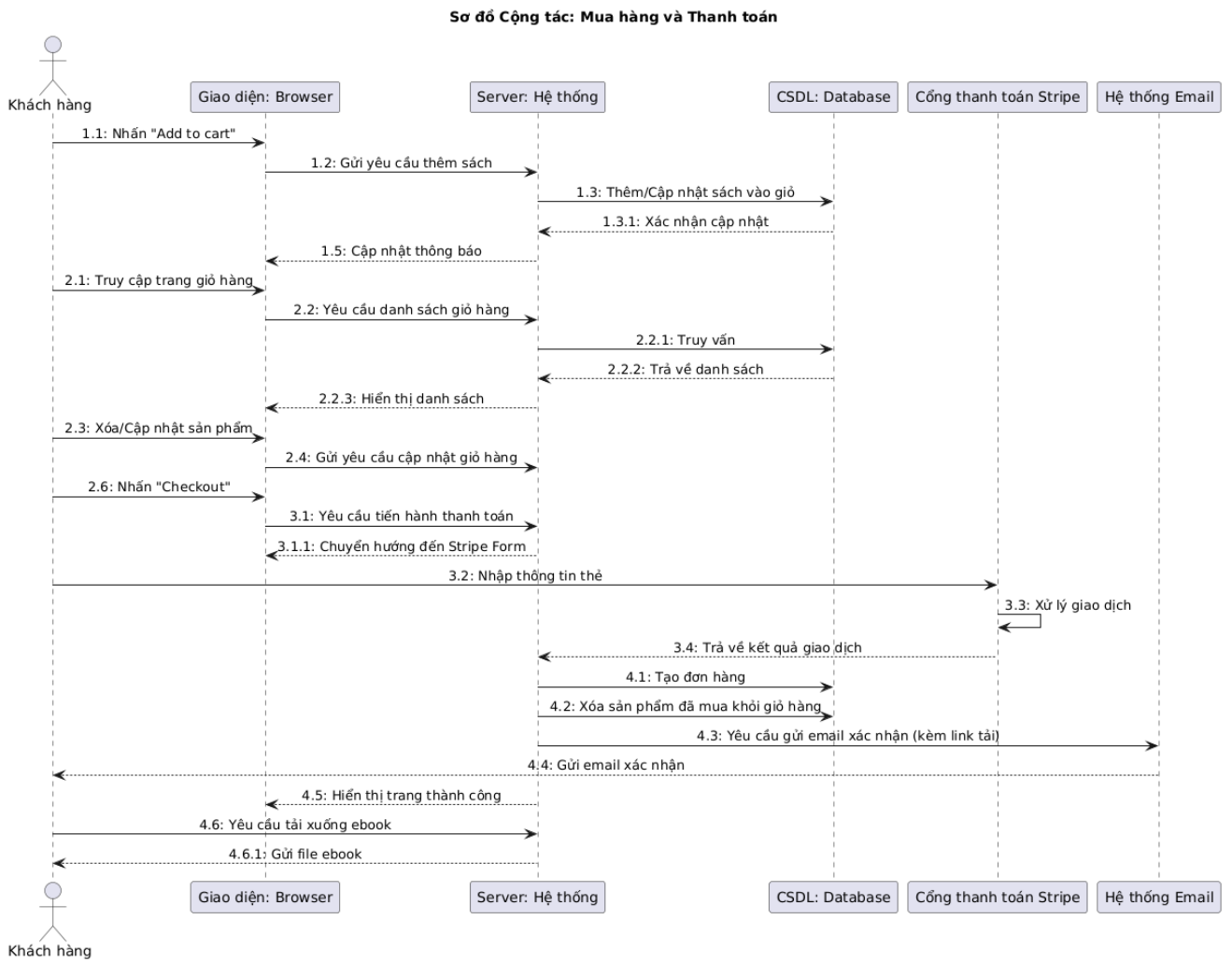
Hình 3.11 Sơ đồ cộng tác: Mua hàng và Thanh Toán
