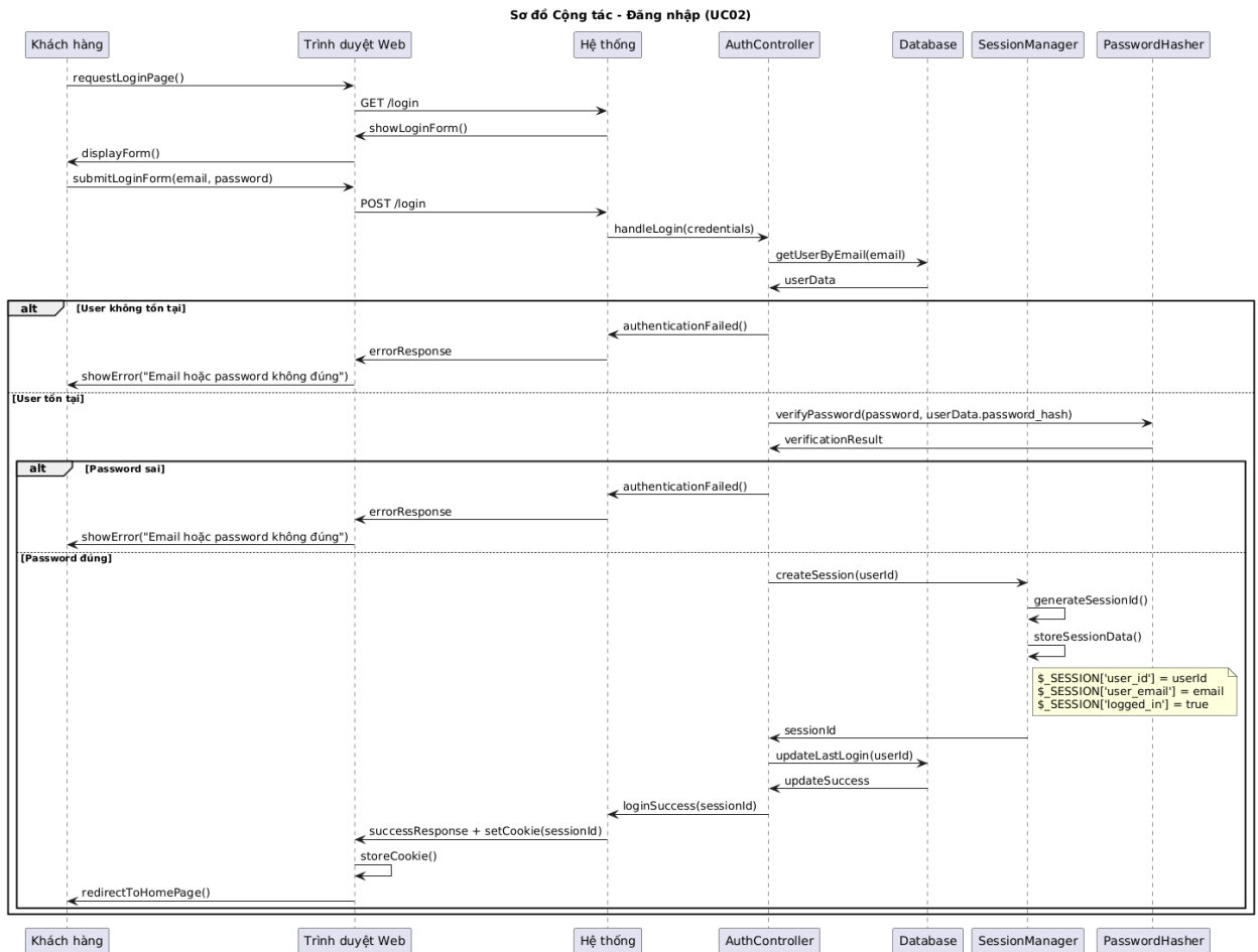
Hình 3.7 Sơ đồ cộng tác - Đăng nhập
